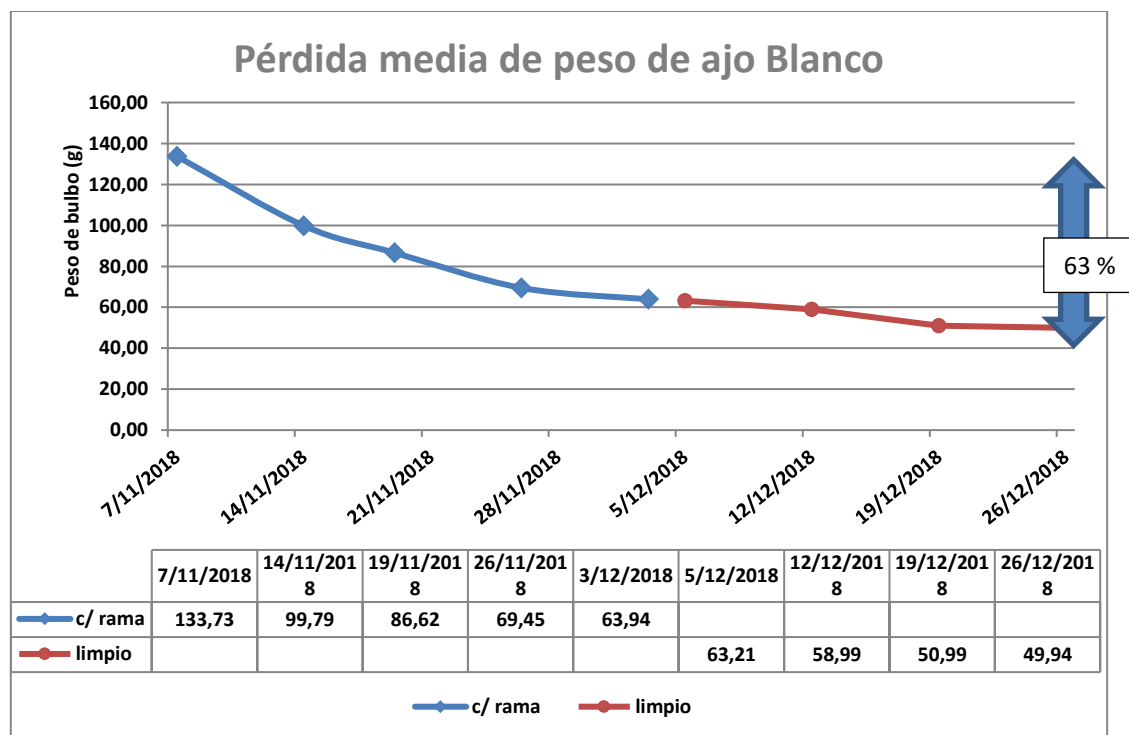
Figura 2 – Pérdida media de peso de bulbo de ajo Blanco. Campaña 2018-2019
